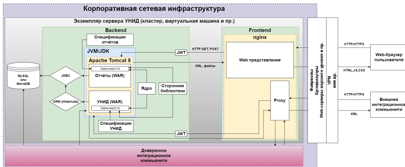
Рис.1. Общая схема приложения, составляющие, их взаимодействие
